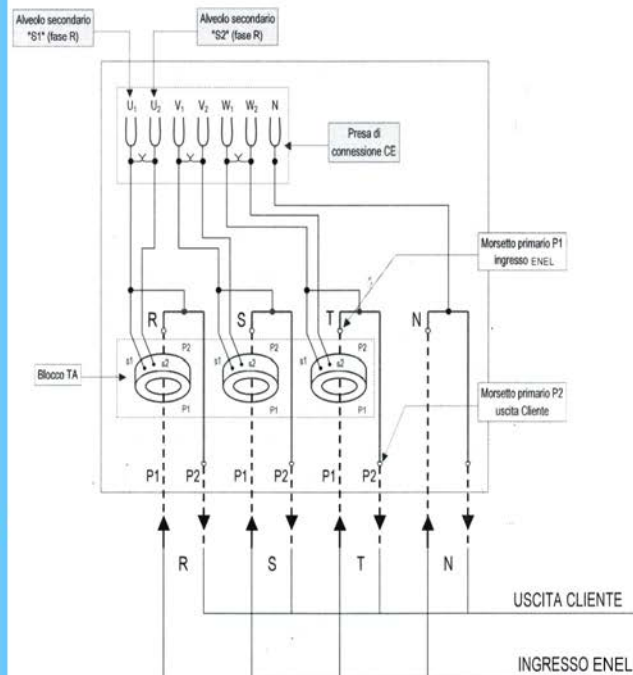
- CABLAGGIO COMPLESSO TA -
